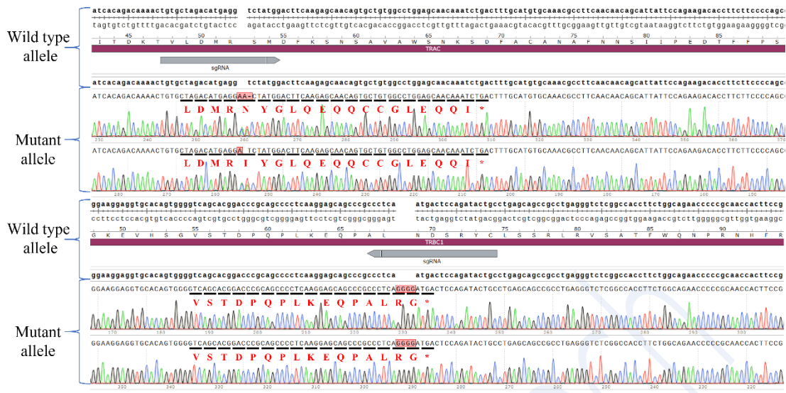
Fig 2. 测序验证 TCR 敲除结果
